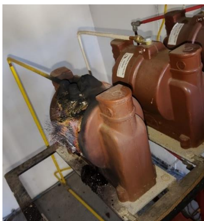
Foto 5: TP (transformador de potencial) avariado.
